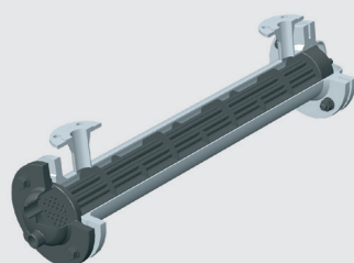
Trubkové výměníky
