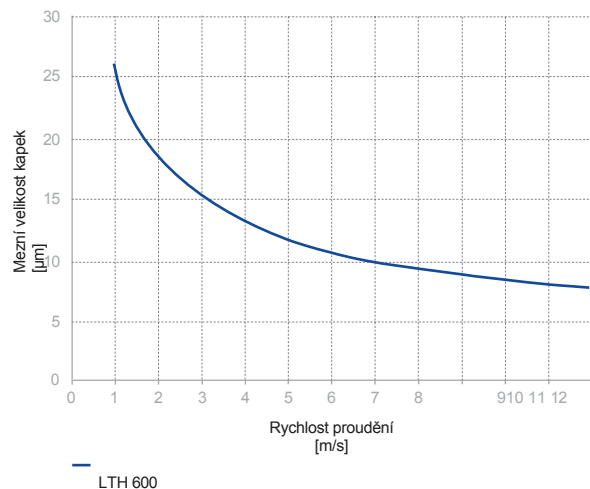
Hraniční diagram kapek LTH 600
