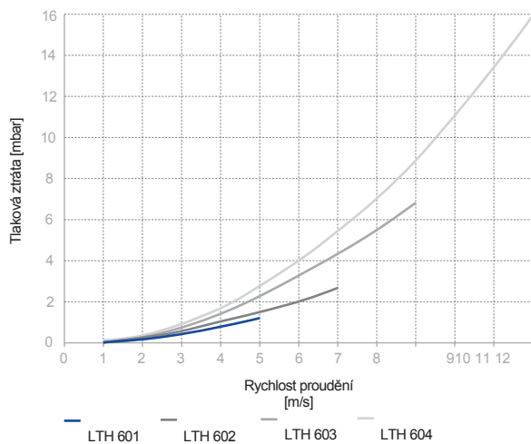
Diagram tlakových ztrát LTH 600
